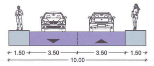
SECȚIUNE A-A' - Str. Cap. Grigore Marin - scara 1:100
