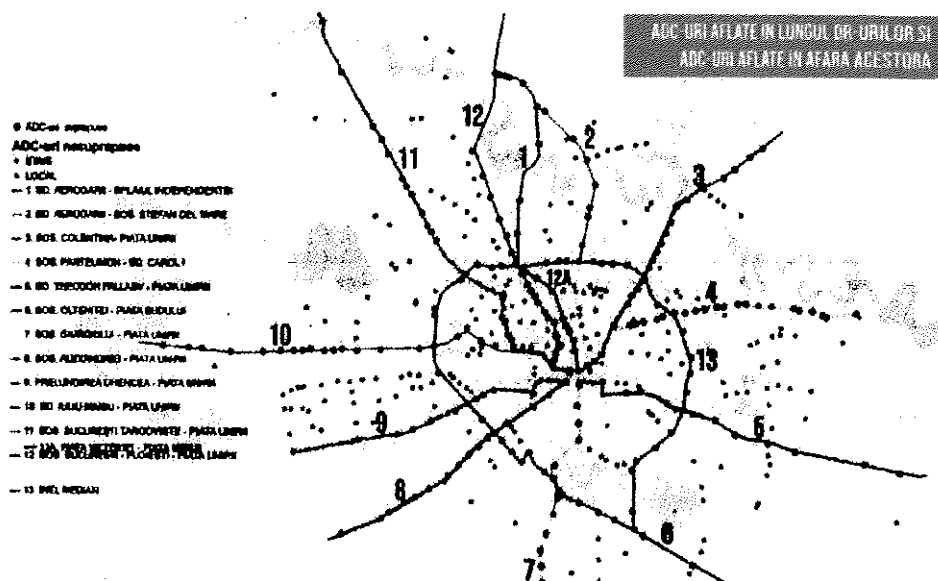
Figura 5. Principalele axe de circulație (1-12) și inelul principal (13)
