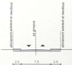
Profil existent A-A' - Calea Serban Voda
